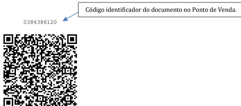
Figura 5 - QRCode
